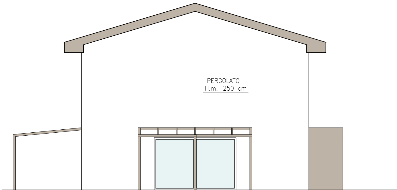
PROSPETTO OVEST
