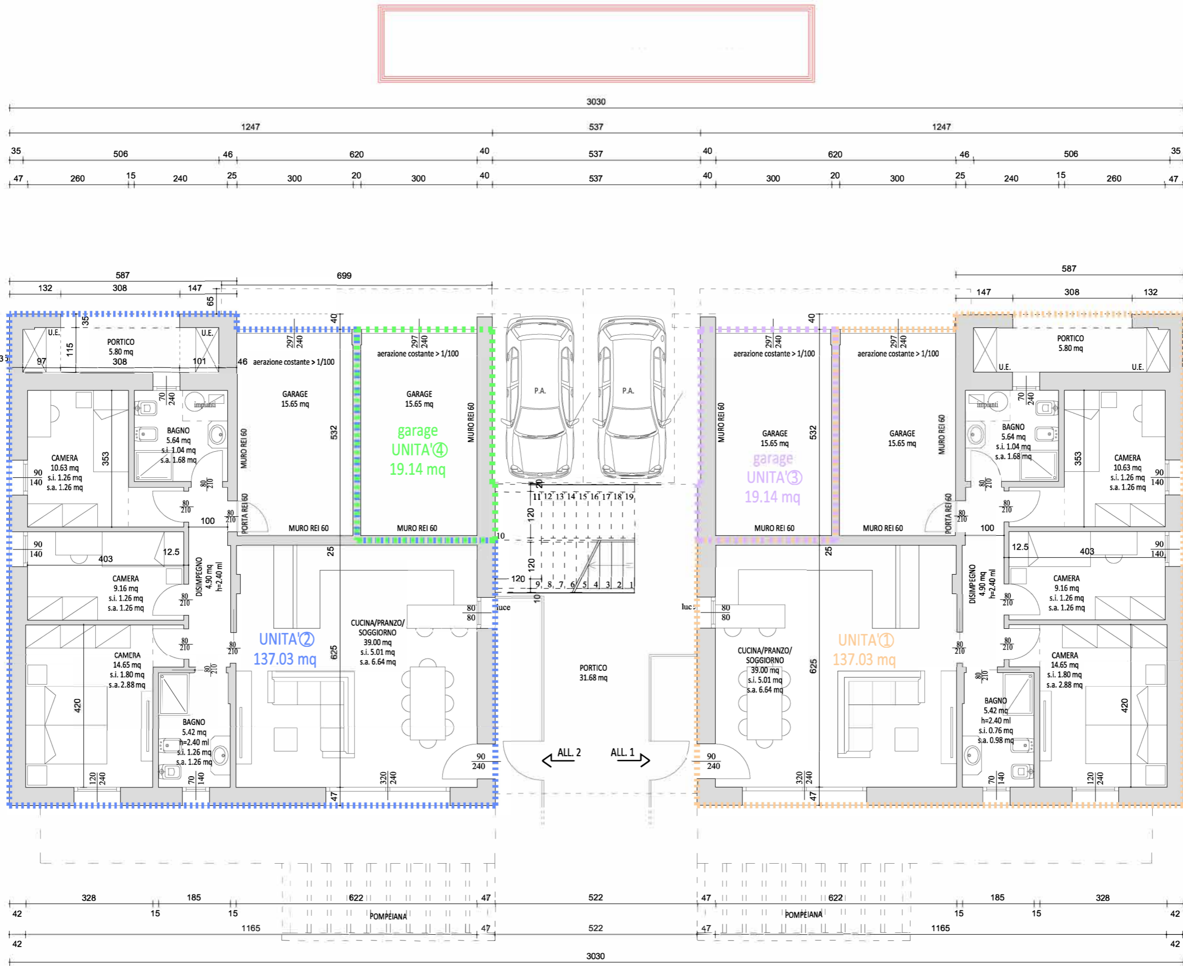
PIANTA PIANO TERRA - SC. 1:50
