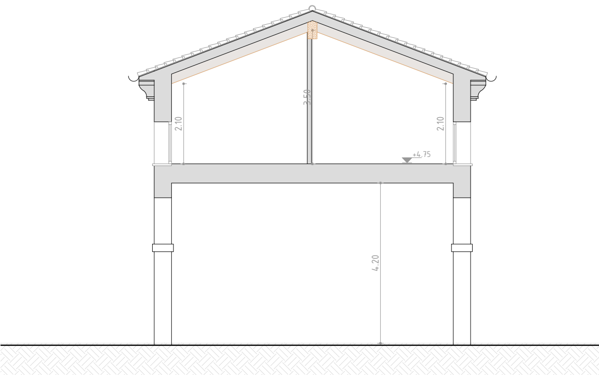
SEZIONE C-C
