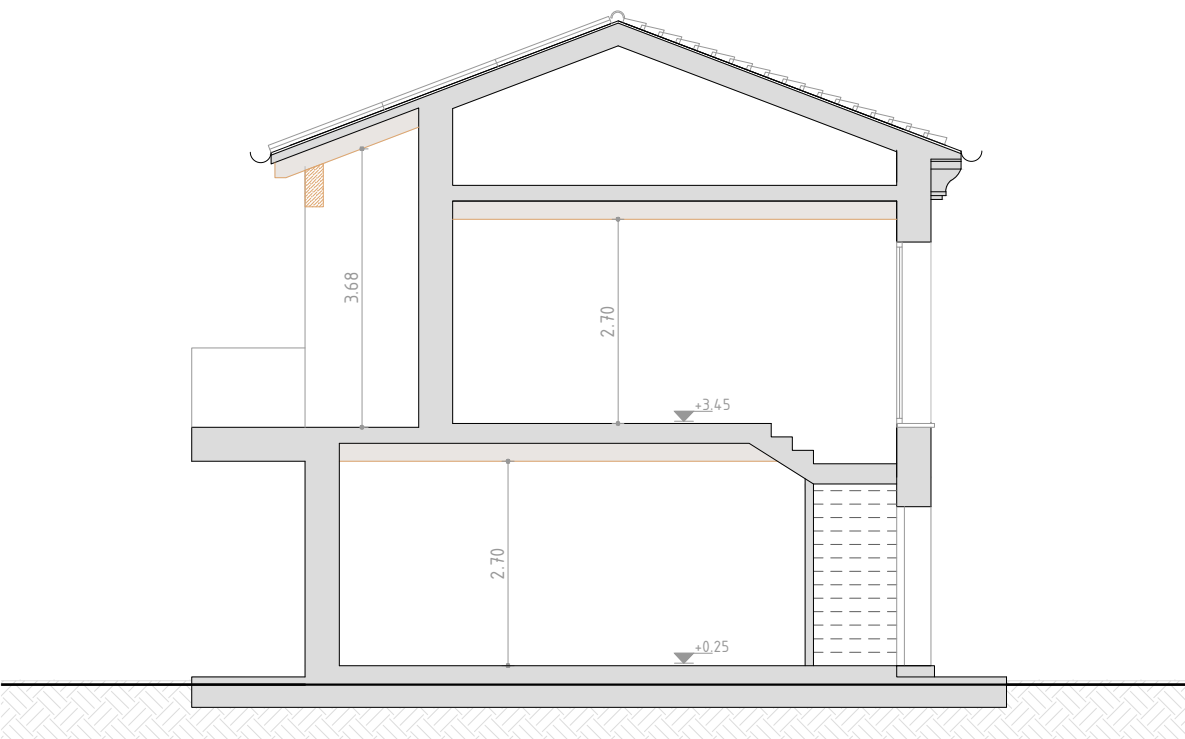
SEZIONE D-D
