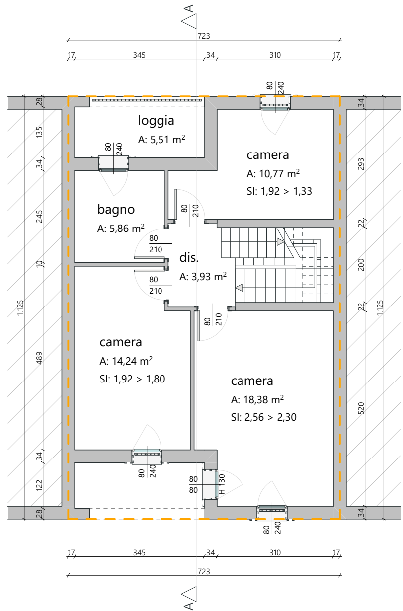
SdF piano primo 1:100
