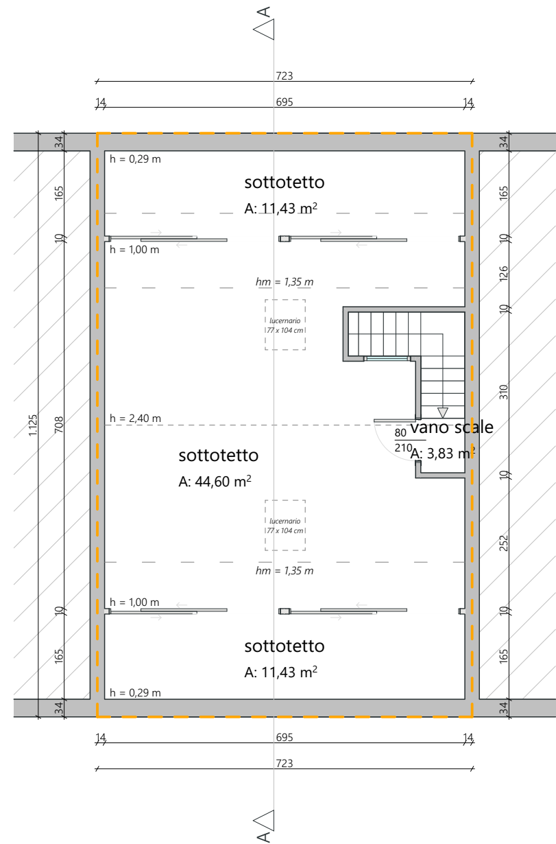
SdF sottotetto 1:100
