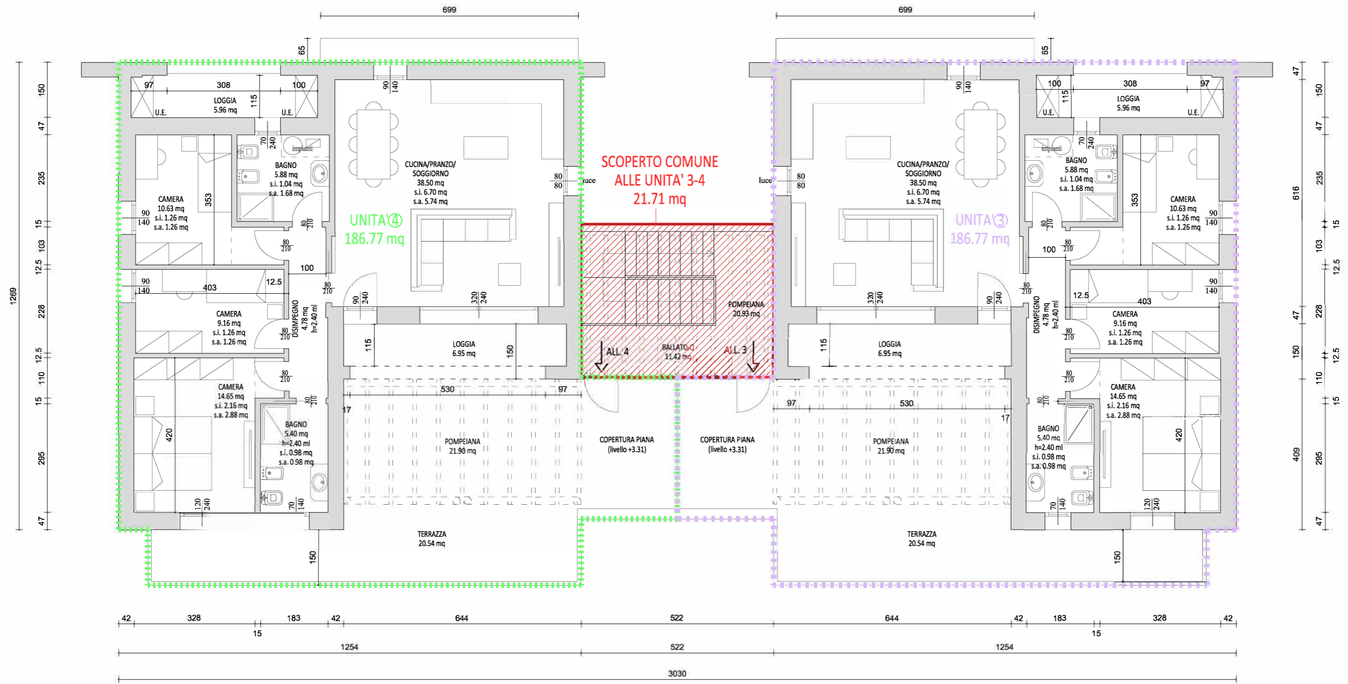
PIANTA PIANO PRIMO - SC. 1:100
