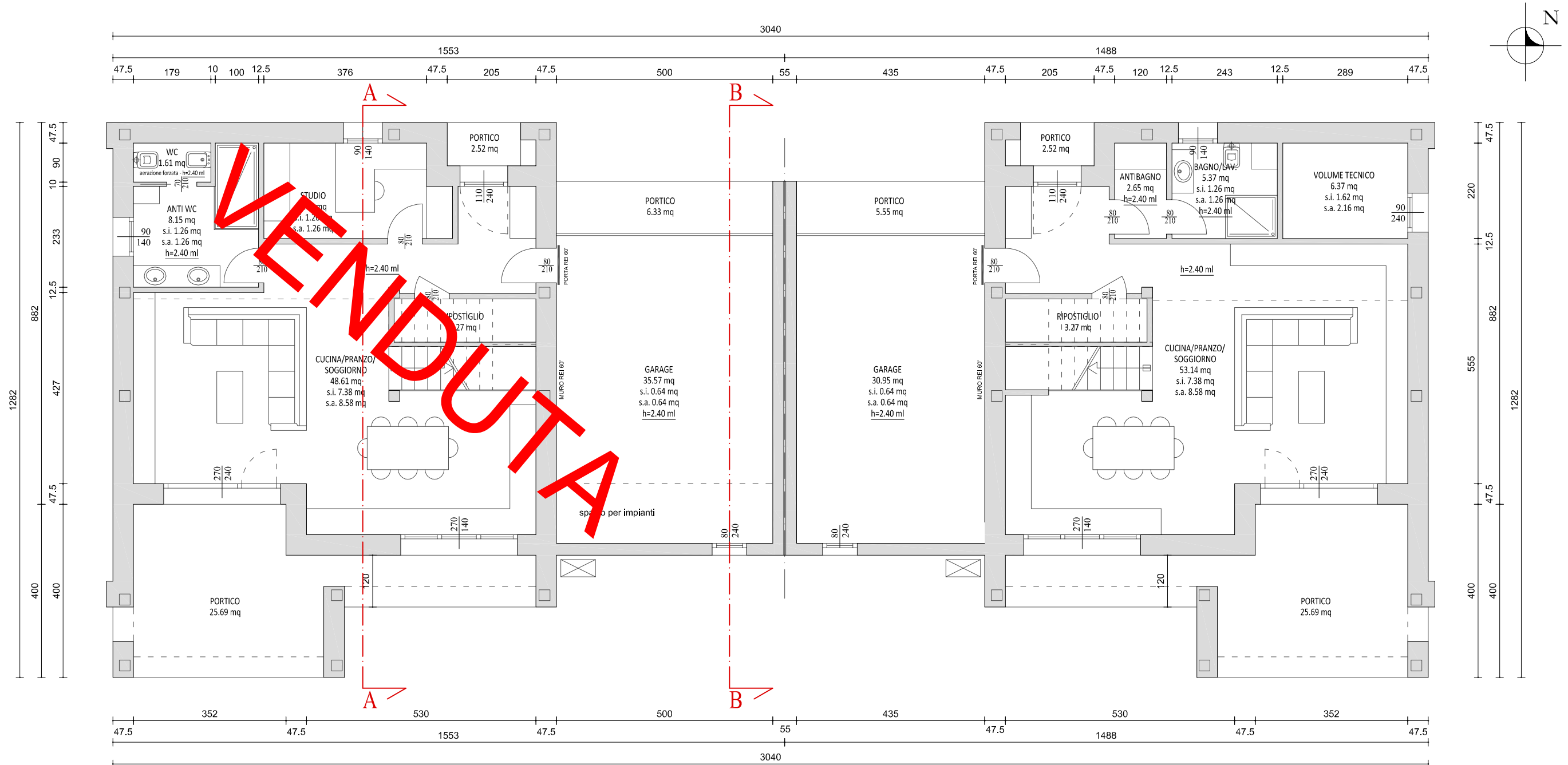
PIANTA PIANO TERRA - SC. 1:100
