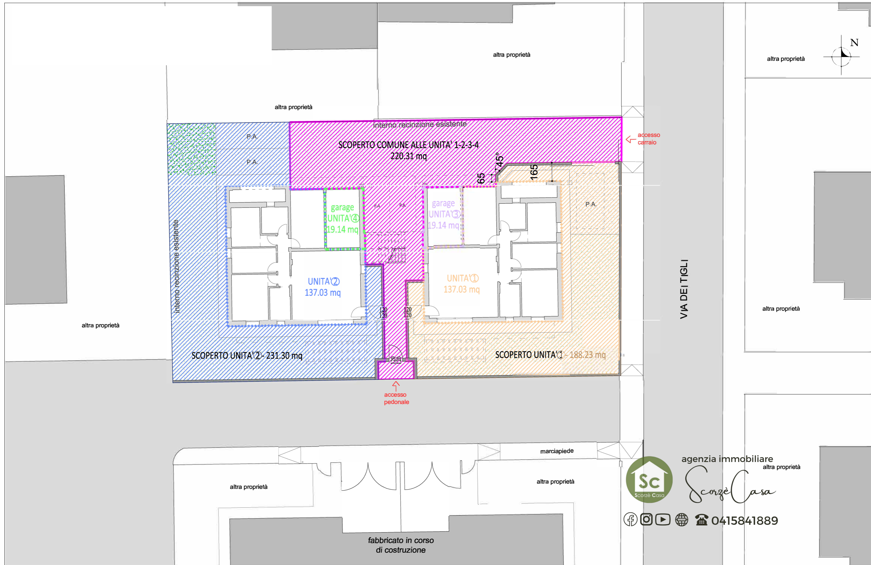
PLANIMETRIA DI PROGETTO - SC. 1:200
