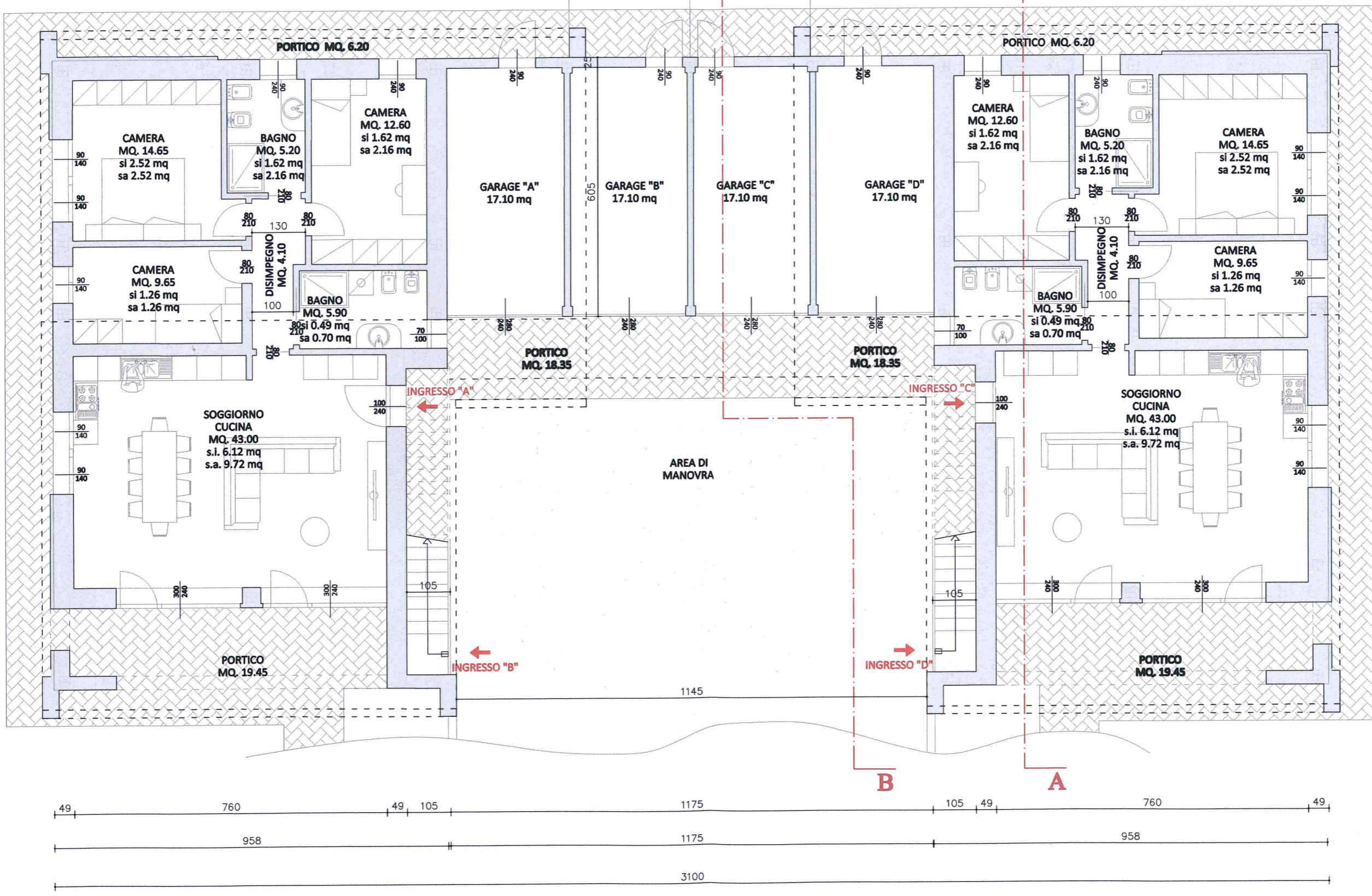
PIANTA PIANO TERRA - SC. 1:100
